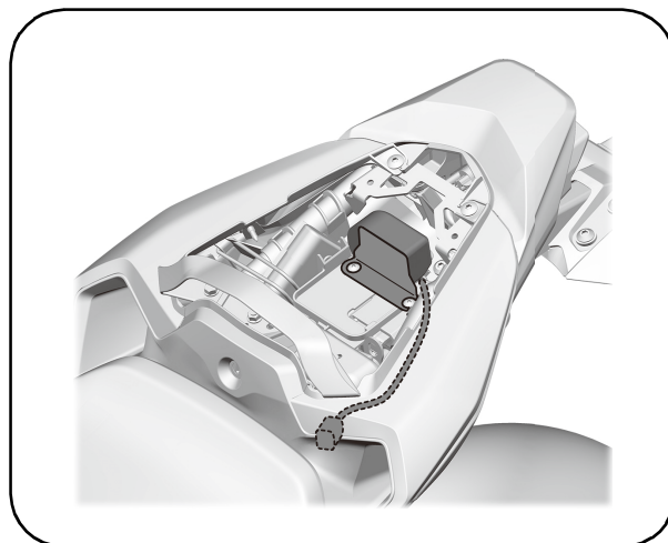
IMAGE D'INSTALLATION
